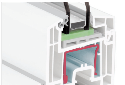
Površinsko zamaknjena izvedba krila
